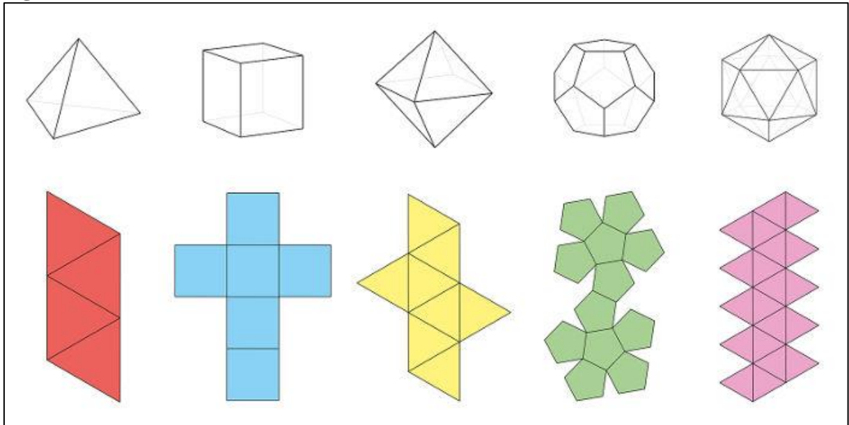
Figura 10 – Poliedros Platônicos.
