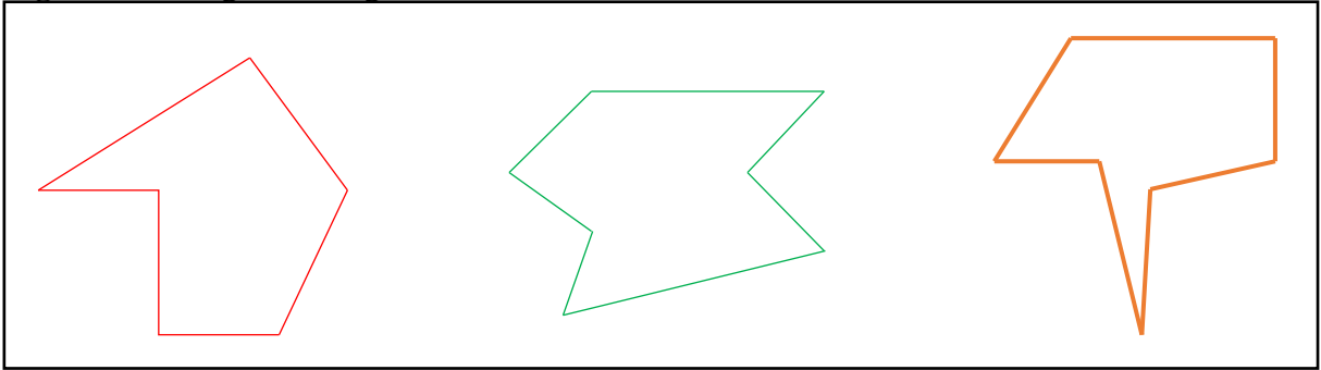
Figura 5 – Polígonos Irregulares.
