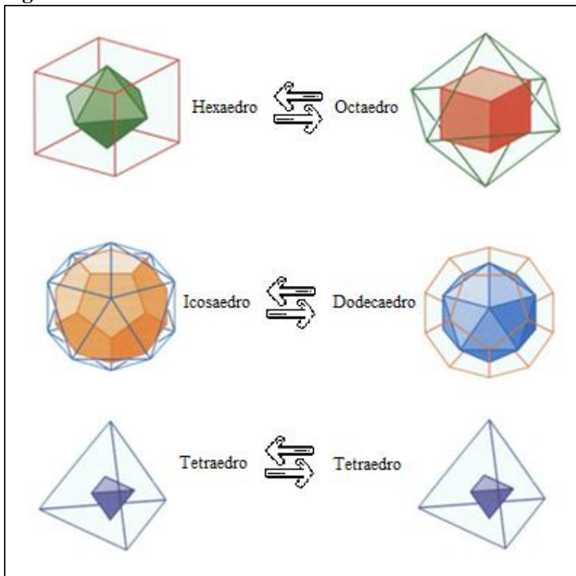
Figura 11 – Poliedros Duais.
