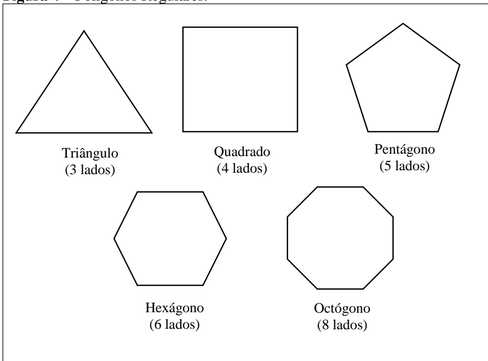
Figura 4 – Polígonos Regulares.
